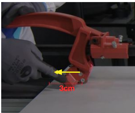
Imagem 54: Primeiro faça um risco com a vîdea de 3cm na extremidade da peça.
