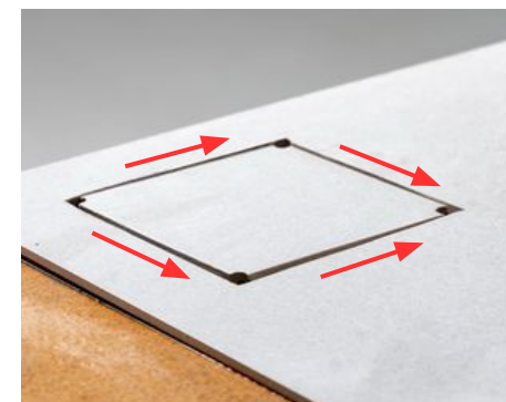
Imagen 83: El corte debe realizarse en dirección a la parte de la pieza con mayor área.
