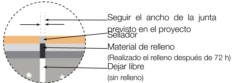
Detalle 04
