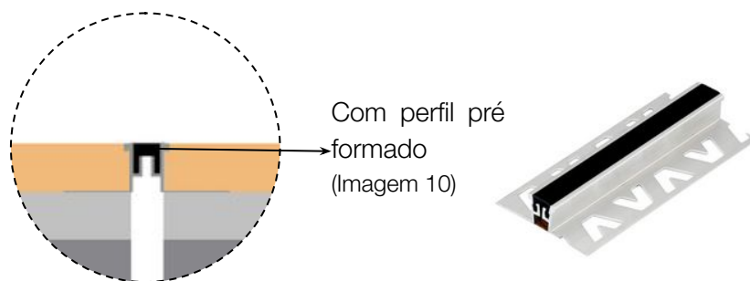
Detalhamento 05
