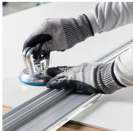
Imagem 71: Fixar o trilho com ventosa na peça.
