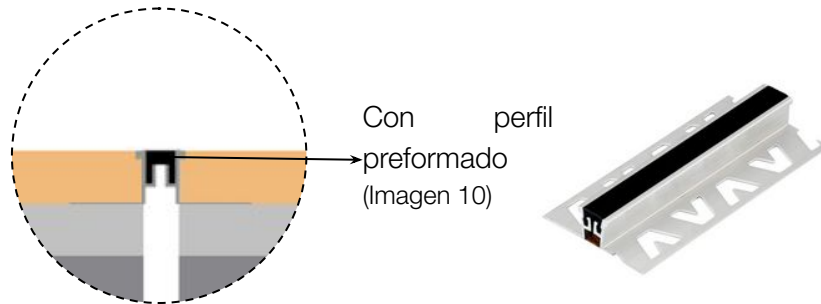
Detalle 05
