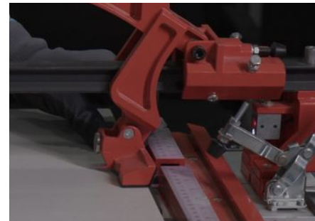
Imagen 56: Coloque la zapata del rayador al inicio de la pieza aplicando presión.
