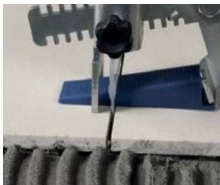
Imagen 43: Realice el ajuste con alicates de presión.
