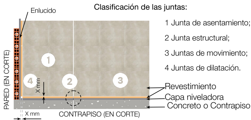
Detalle 01
