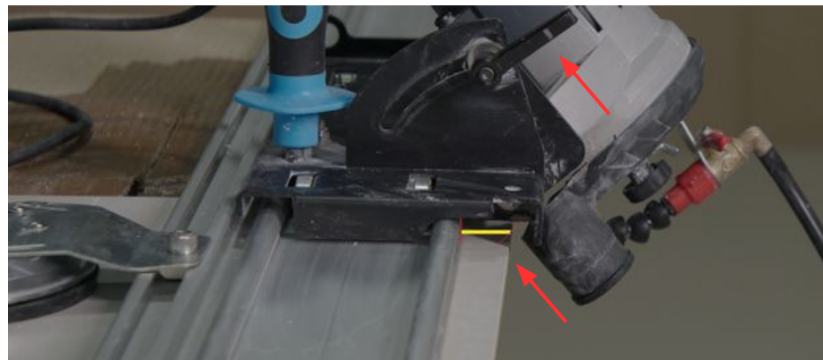
Imagem 96: Ferramenta sobre o trilho e ajuste da angulação do corte com alavanca.
