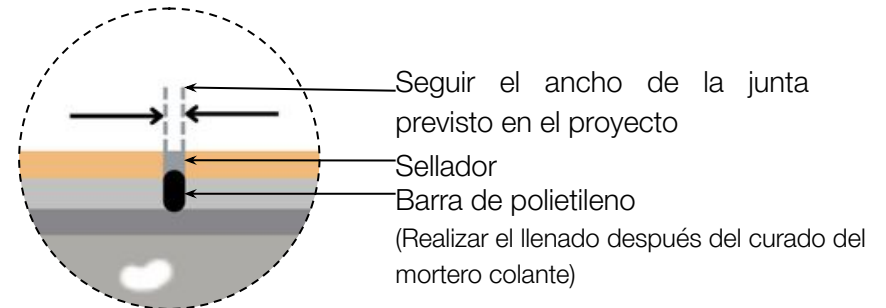
Detalle 02
