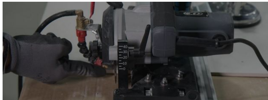
Imagen 74: Ajuste la palanca según la profundidad de corte.
