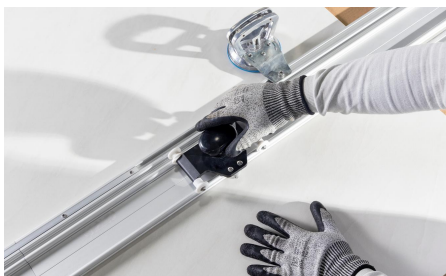
Imagen 62: Coloque la rueda guía sobre el riel
