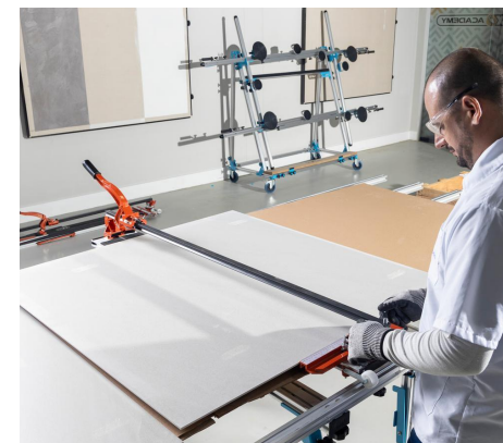
Imagem 51: Encaixa da peça estabilizada sobre o riscador.
