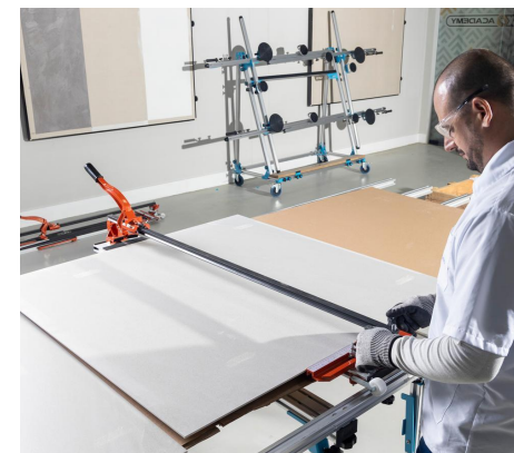
Imagen 51: Encaje de la pieza estabilizada sobre el rayador.
