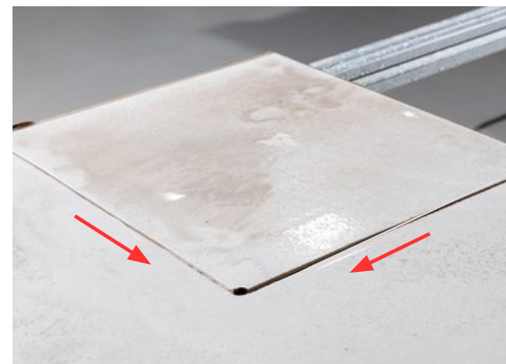
Imagen 88: El corte debe realizarse en dirección a la parte de la pieza con mayor área.
