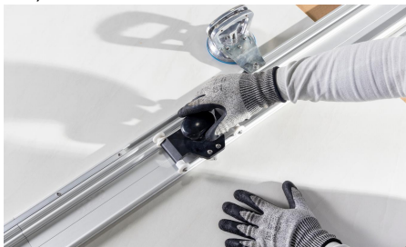
Imagem 62: Encaixe o rodel sobre o trilho
