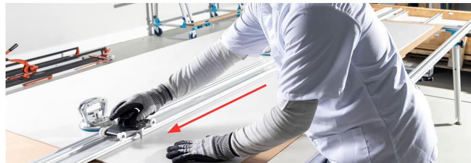
Imagem 64: Deslize o rodel com riscador diamantado sobre o local do corte.
