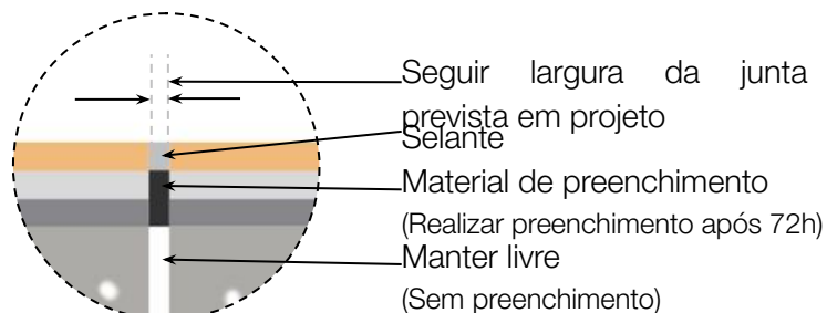
Detalhamento 04
