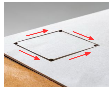
Imagen 83: El corte debe realizarse en dirección a la parte de la pieza con mayor área.
