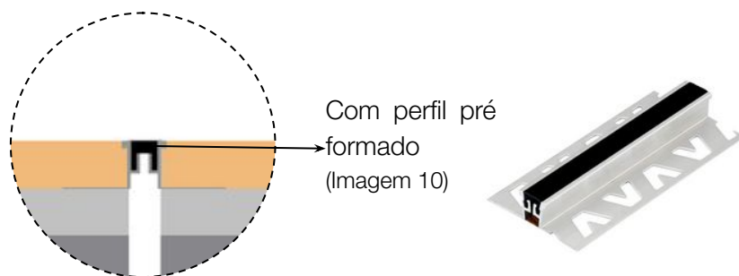
Detalhamento 05
