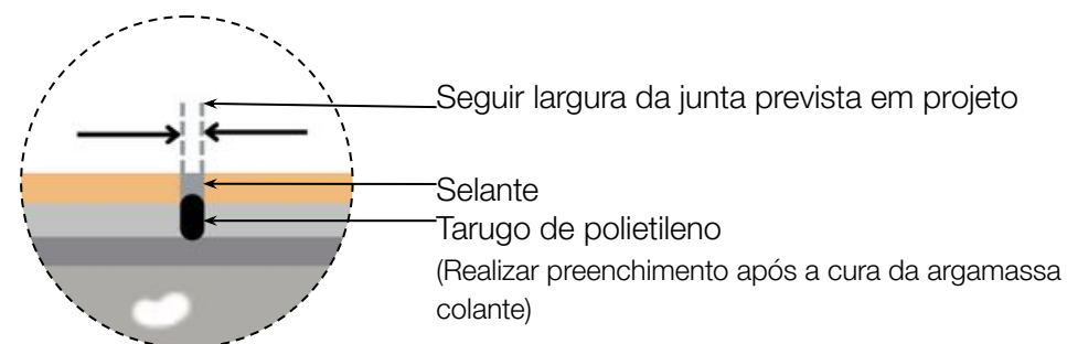
Detalhamento 02
