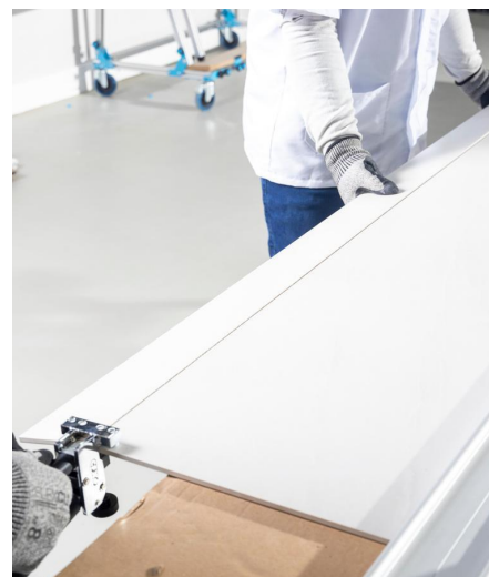
Imagem 68: Na outra extremidade da peça gire a manivela do alicate para a abertura parcial, por fim faça pressão manual no centro da peça.
