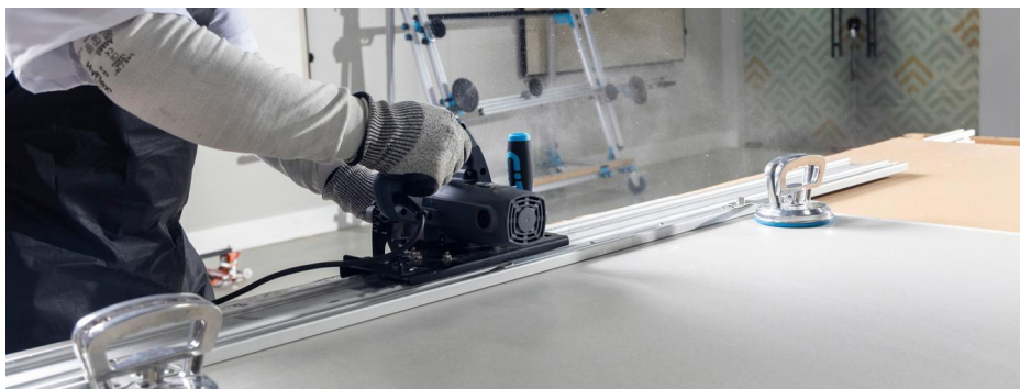
Imagen 77: Deslice la sierra de porcelanato sobre el riel, sin forzar el avance del disco sobre la pieza.
