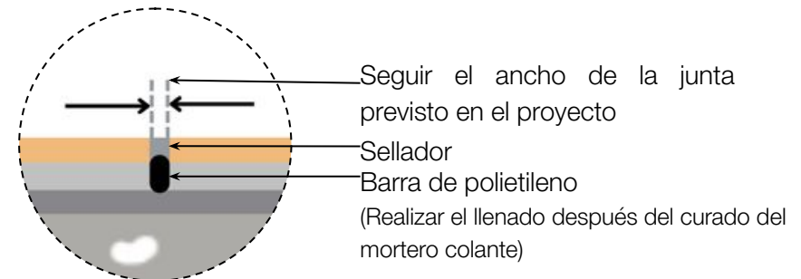
Detalle 02
